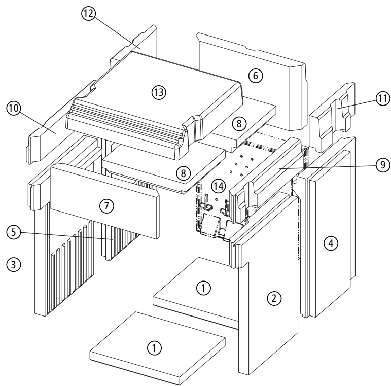
Abb. 5.4 Ersatzteile Feuerraumauskleidung DIAMANT H13.2
