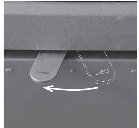
Abb. 4.17 Luftschieber ganz links, Verbrennungsluft geschlossen
