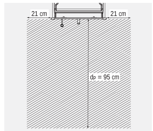
Abb. 2.3 Strahlungsbereich der Gerätefront bei DIAMANT H13.2 – schematische Darstellung
