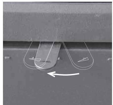
Abb. 4.16 Luftschieber ca. 1/4 geöffnet (25%), Betriebsstellung bei Nennwärmeleistung
