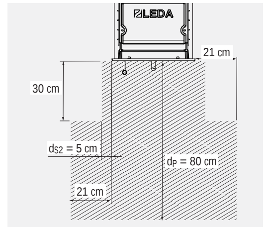
Abb. 2.2 Strahlungsbereich der Gerätefront bei DIAMANT H10.2 und DIAMANT H20.2 – schematische Darstellung
