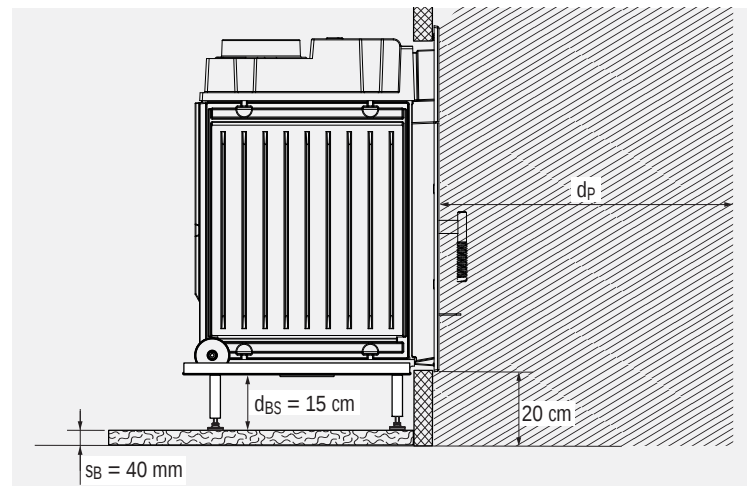
Abb. 2.4 Strahlungsbereich der Front – schematische Darstellung Seitenansicht
