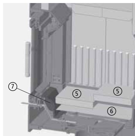
Abb. 4.25 Bodensteine, Bodenblech und Revisionsdeckel
