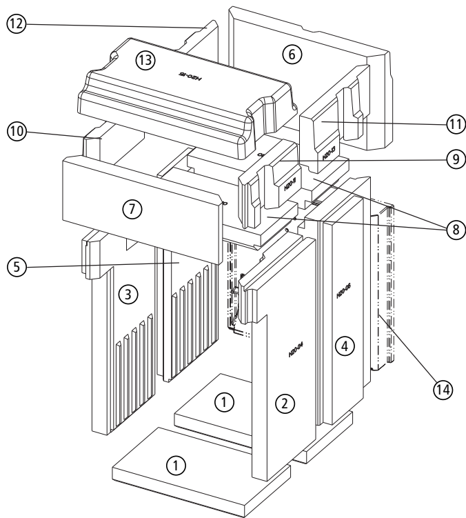
Abb. 5.3 Ersatzteile Feuerraumauskleidung DIAMANT H20.2
