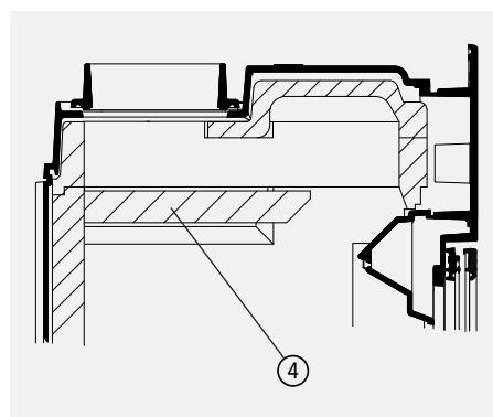
Abb. 4.24 Umlenkung im Feuerraum des DIAMANT
