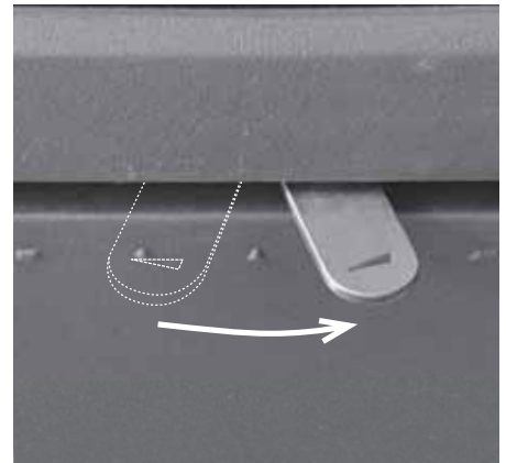
Abb. 4.19 Luftschieber ganz rechts, Anheizstellung und Betriebsstellung bei Speicherleistung
