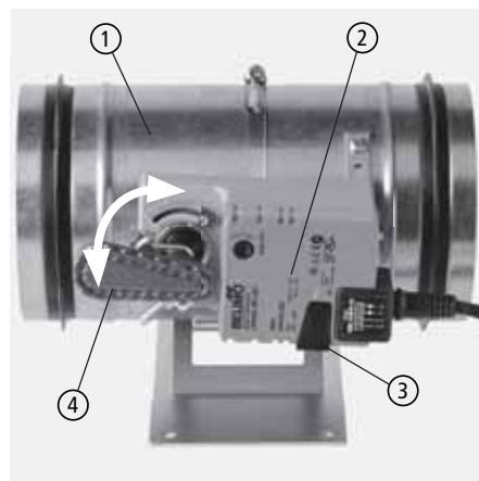
Abb. 4.22 Verbrennungsluftklappe mit Stellmotor
