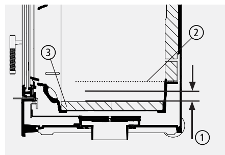
Abb. 4.23 Aschebett, Ascheniveau
