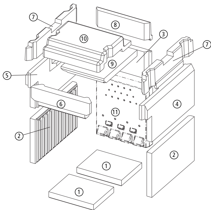
Abb. 5.2 Ersatzteile Feuerraumauskleidung DIAMANT H10.2
