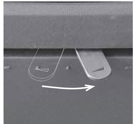
Abb. 4.15 Luftschieber ganz rechts, Anheizstellung
