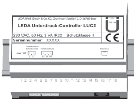
Abb. 10.1 Geräte Kennzeichnung auf der Schalteinheit des LUC
