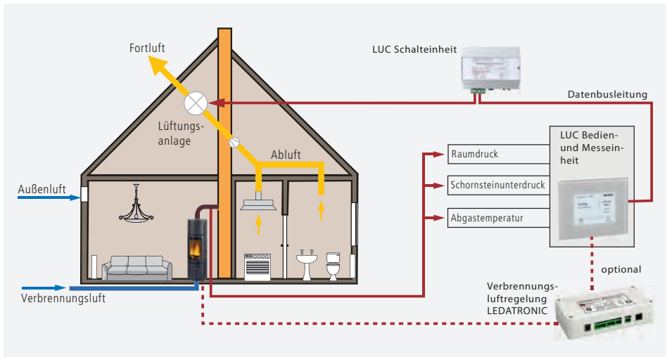
Abb. 3.1 Systemdarstellung, Feuerstätte, Lüftungsanlage, optional LT3 zusammen mit LUC
