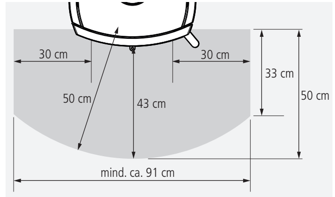
Nicht brennbarer Belag vor der Feuerraumöffnung
