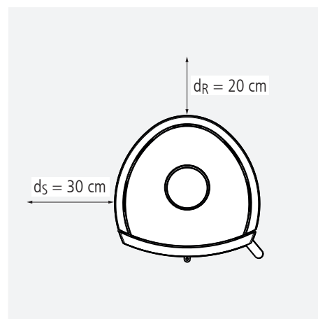
DELTA W: Mindestabstände zu brennbaren Baustoffen oder Bauteilen
