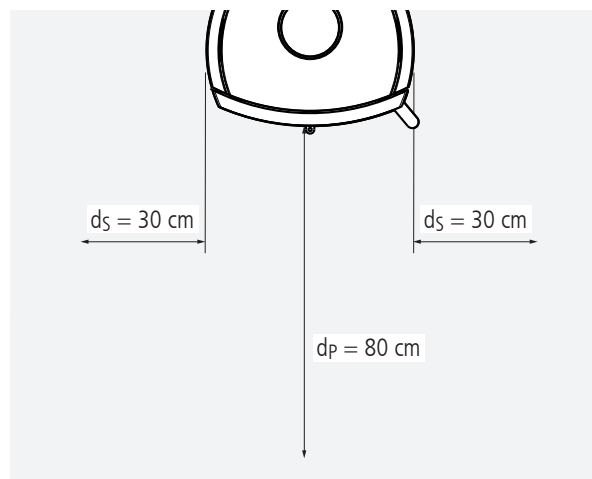
DELTA W: Mindestabstände im Bereich der Sichtscheibe – schematische Darstellung
