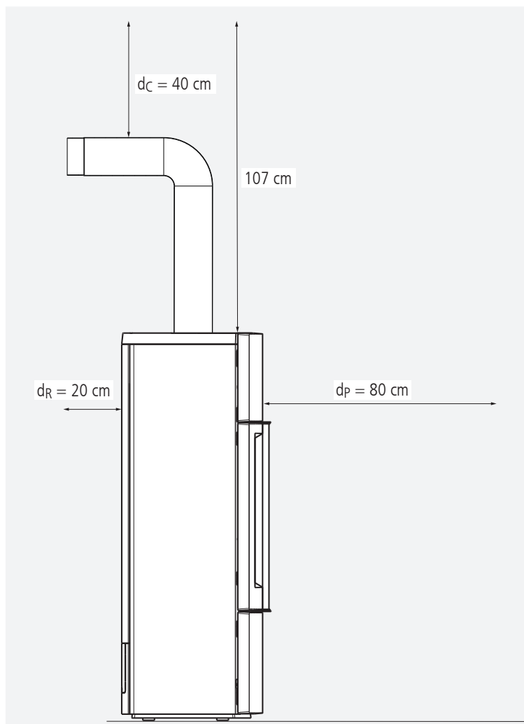
DELTA W: Strahlungsbereich der Sichtscheibe – schematische Darstellung, Seitenansicht
