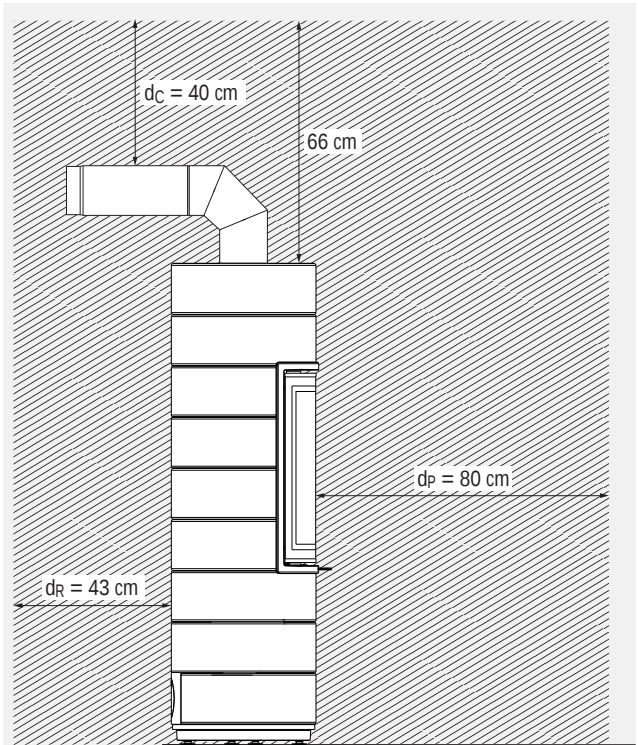
Abb. 2.3 Strahlungsbereich der Sichtscheibe – schematische Darstellung, Seitenansicht
