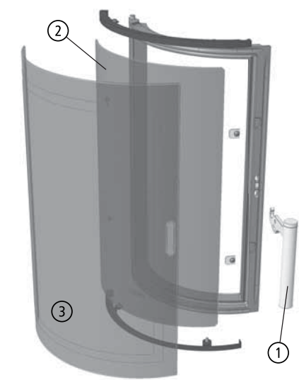
Abb. 5.1 Ersatzteilübersicht – Feuertür
