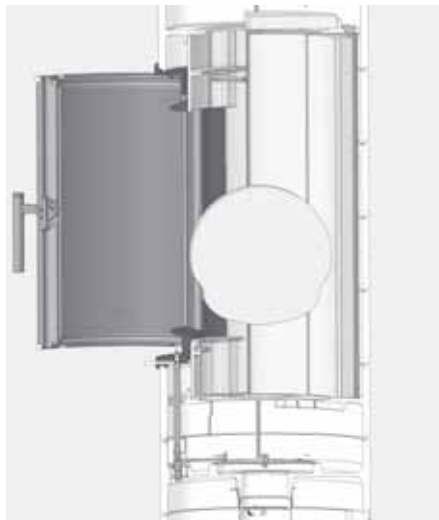
Abb. 4.38 Drehen des Bodensteins im Brennraum und Entnehmen
