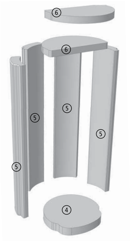
Abb. 5.2 Ersatzteilübersicht – Feuerraumauskleidung
