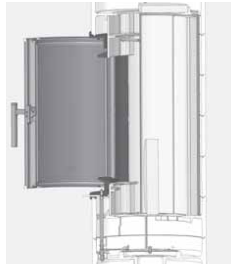
Abb. 4.37 Aufrichten des Bodensteins im Brennraum
