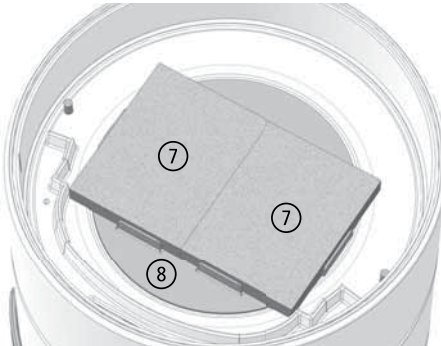
Abb. 5.3 Ersatzteilübersicht – Katalysator
