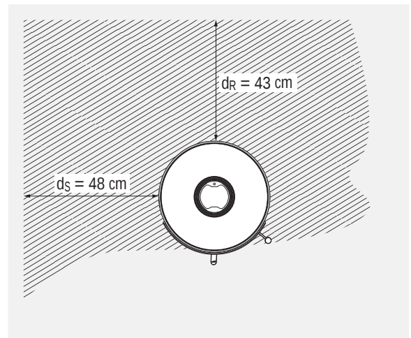
Abb. 2.4 Mindestabstände zu brennbaren Baustoffen oder Bauteilen
