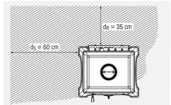
Abb. 2.5 Mindestabstände zu brennbaren Baustoffen oder Bauteilen
