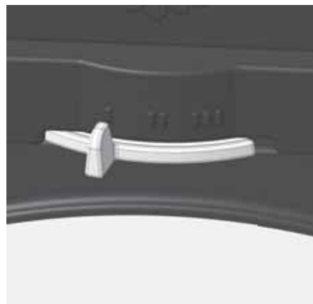
Abb. 4.15 Verbrennungsluftschieber ganz links, Markierung „I“, Verbrennungsluft geschlossen
