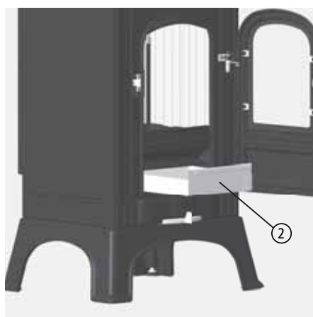
Abb. 4.36 Aschekasten entnehmen
