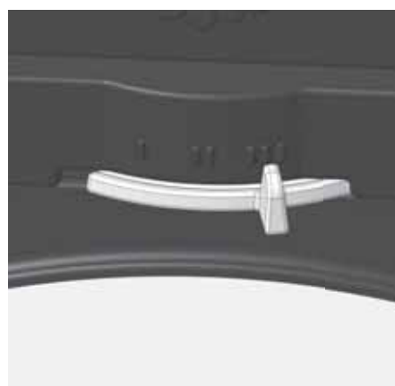
Abb. 4.16 Verbrennungsluftschieber ganz rechts, Markierung „III“, Verbrennungsluft komplett geöffnet, Anheizen
