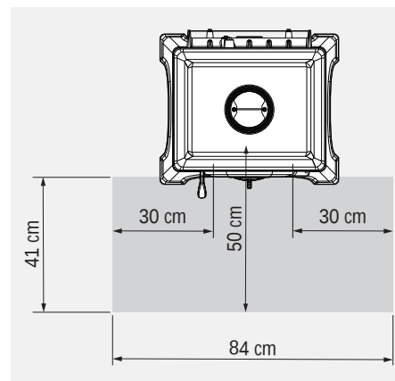
Abb. 2.1 Nicht brennbarer Belag vor der Feuerraumöffnung
