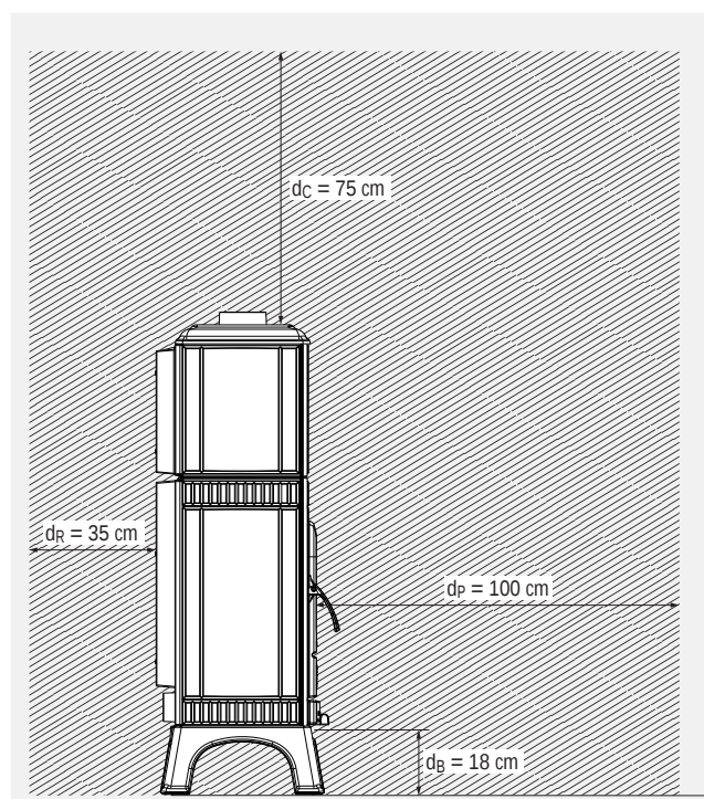
Abb. 2.3 Strahlungsbereich der Sichtscheibe – schematische Darstellung, Seitenansicht – EDDA plus oder EDDA tea
