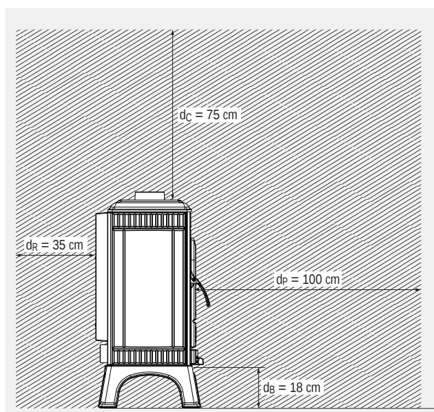
Abb. 2.4 Strahlungsbereich der Sichtscheibe – schematische Darstellung, Seitenansicht – EDDA small
