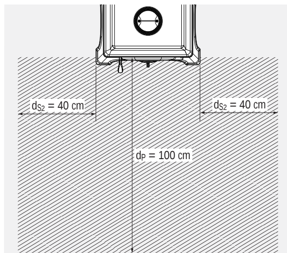
Abb. 2.2 Mindestabstände im Bereich der Sichtscheibe
