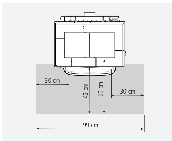
Nicht brennbarer Belag vor den Feuerraumöffnungen bei eingesetzter Türsicherung in der seitlichen Befülltür
