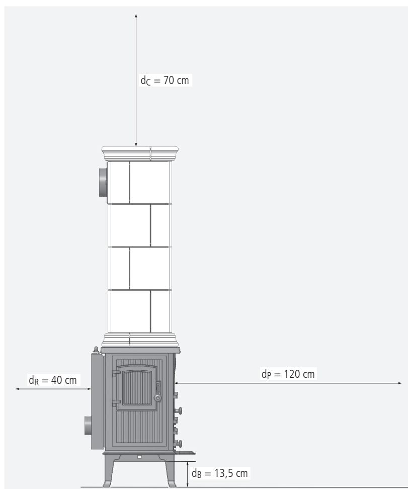
Strahlungsbereich der Sichtscheibe – schematische Darstellung, Seitenansicht
