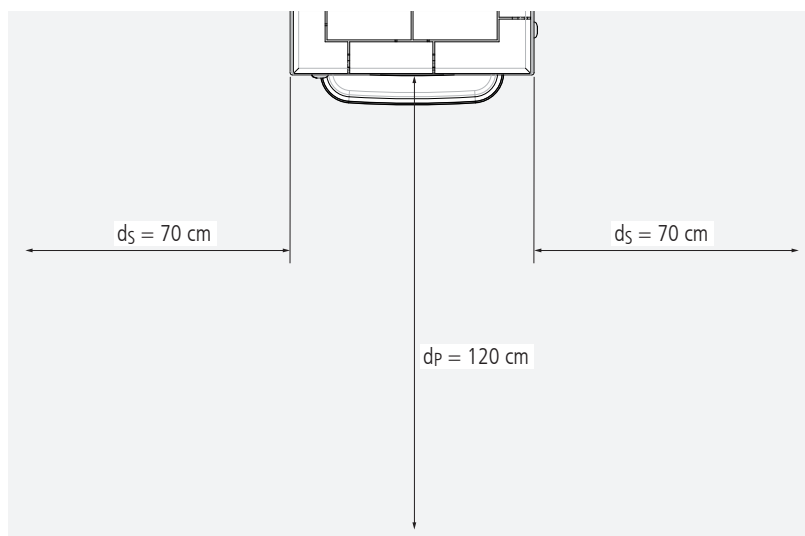
Mindestabstände im Strahlungsbereich der Sichtscheibe / im Bereich der Front
