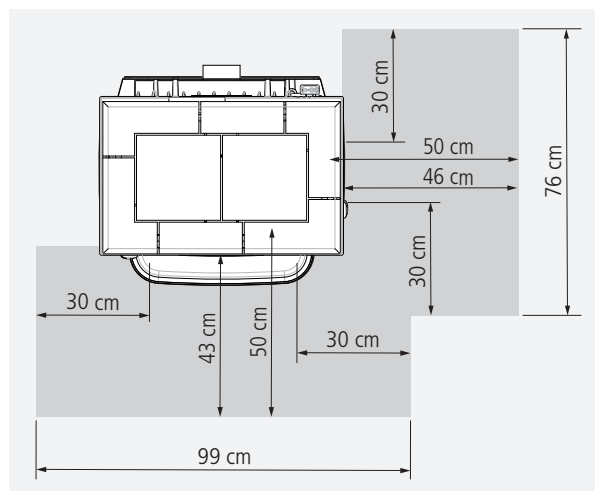
Nicht brennbarer Belag vor der Feuerraumöffnung
