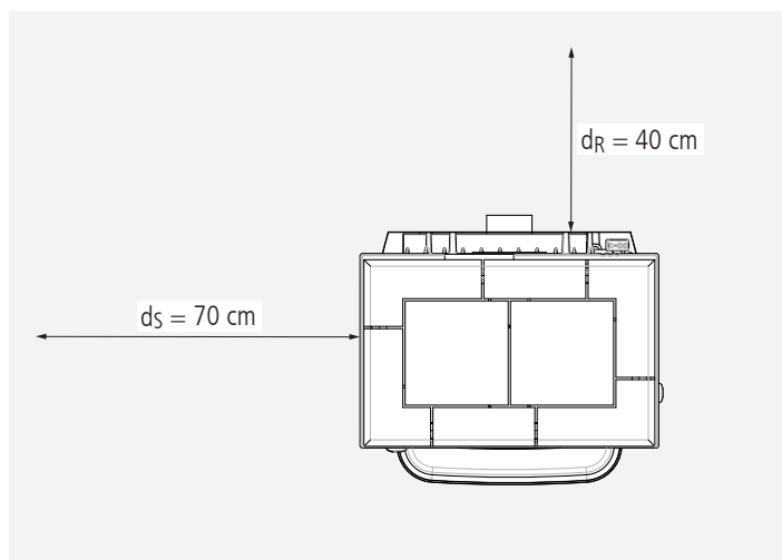
Mindestabstände zu brennbaren Materialien hinten und seitlich
