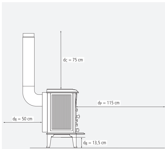
Strahlungsbereich der Sichtscheibe – schematische Darstellung, Seitenansicht bei Anschluss hinten
