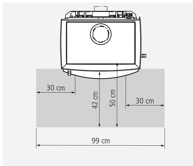
ARUBA: Nicht brennbarer Belag vor den Feuerraumöffnungen bei eingesetzter Türsicherung in der seitlichen Befülltür
