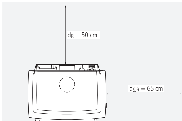
Mindestabstände zu brennbaren Materialien – Abstand hinten und Seitenabstand rechts
