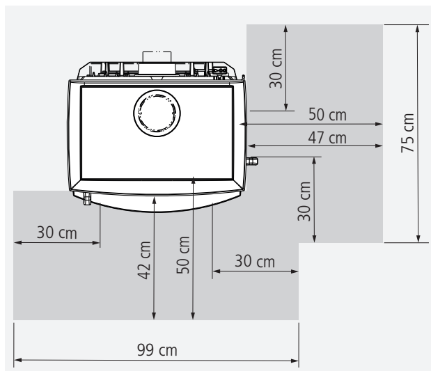
ARUBA: Nicht brennbarer Belag vor den Feuerraumöffnungen
