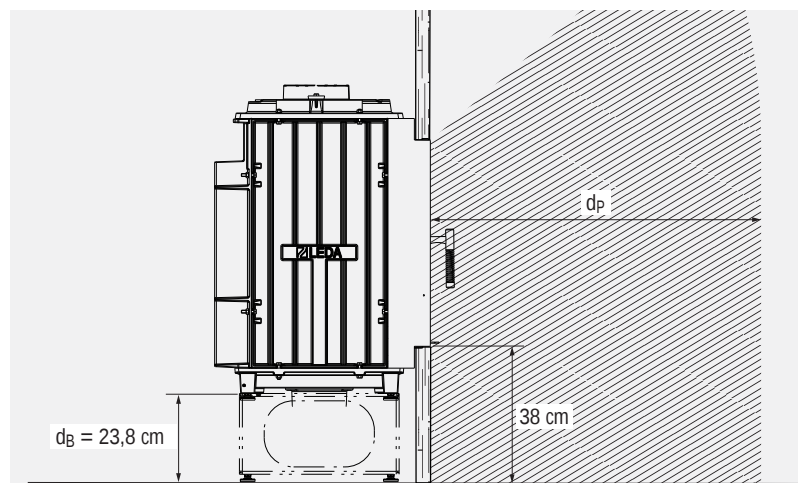
Abb. 2.4 Strahlungsbereich der Front – schematische Darstellung Seitenansicht
