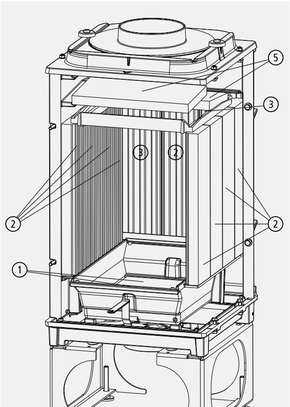
Abb. 5.1 Ausmauerung TURMA F
