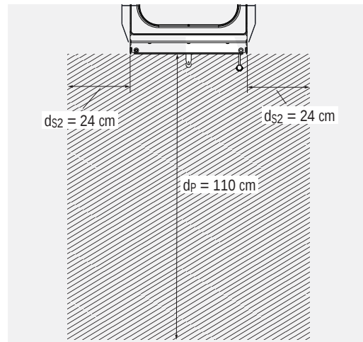
Abb. 2.2 Strahlungsbereich der Gerätefront bei TURMA F, TURMA HL, TURMA XL F und TURMA XL HL – schematische Darstellung
