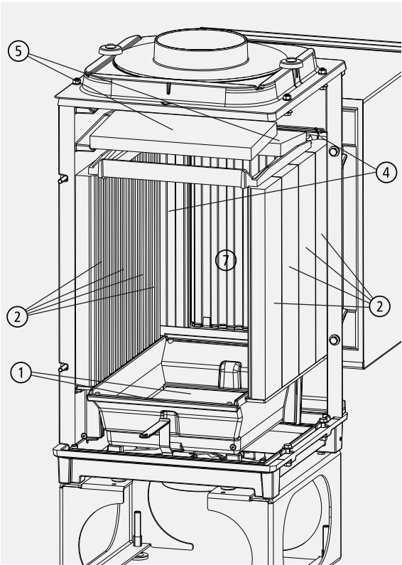
Abb. 5.2 Ausmauerung TURMA HL
