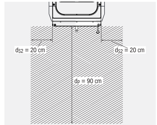
Abb. 2.3 Strahlungsbereich der Gerätefront bei TURMA DS und TURMA XL DS – schematische Darstellung
