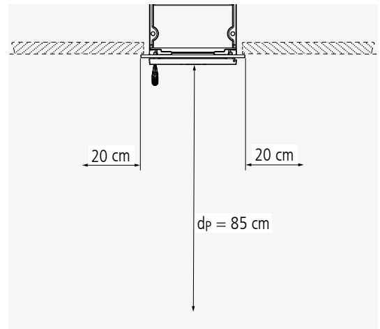
Abb. 2.1 Strahlungsbereich der Gerätefront bei RUBIN K15.2 – schematische Darstellung
