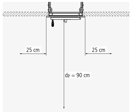
Abb. 2.2 Strahlungsbereich der Gerätefront bei RUBIN K16.2 / RUBIN K17.2 – schematische Darstellung
