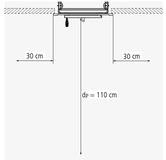
Abb. 2.4 Strahlungsbereich der Gerätefront bei RUBIN K19.2 – schematische Darstellung
