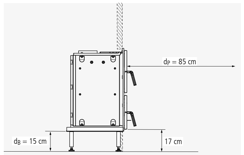
Abb. 2.6 Strahlungsbereich der Front beim RUBIN K15.2 – schematische Darstellung Seitenansicht
