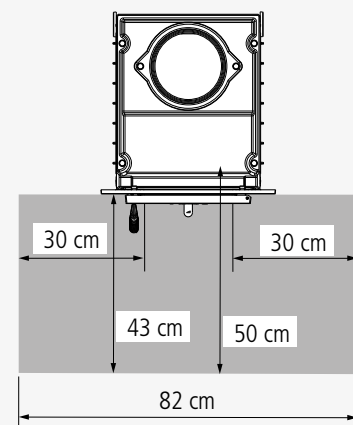
Abb. 2.8 nicht brennbarer Belag vor der Feuerraumöffnung – schematische Darstellung
