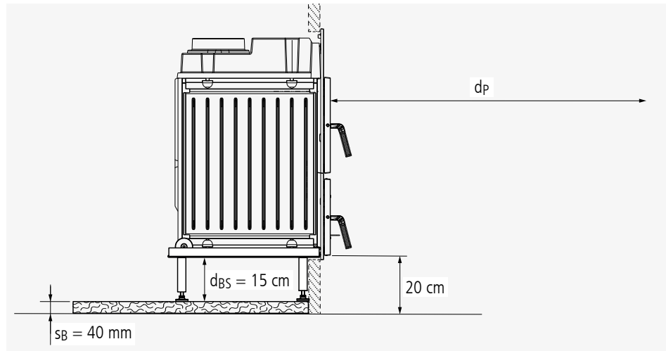
Abb. 2.7 Strahlungsbereich der Front beim RUBIN K16.2 / RUBIN K17.2 / RUBIN K18.2 / RUBIN K19.2 / RUBIN K20.2 / RUBIN K21.2 – schematische Darstellung Seitenansicht
