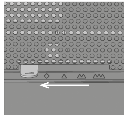
Abb. 4.26 Luftschieber ganz links, Verbrennungsluft geschlossen
