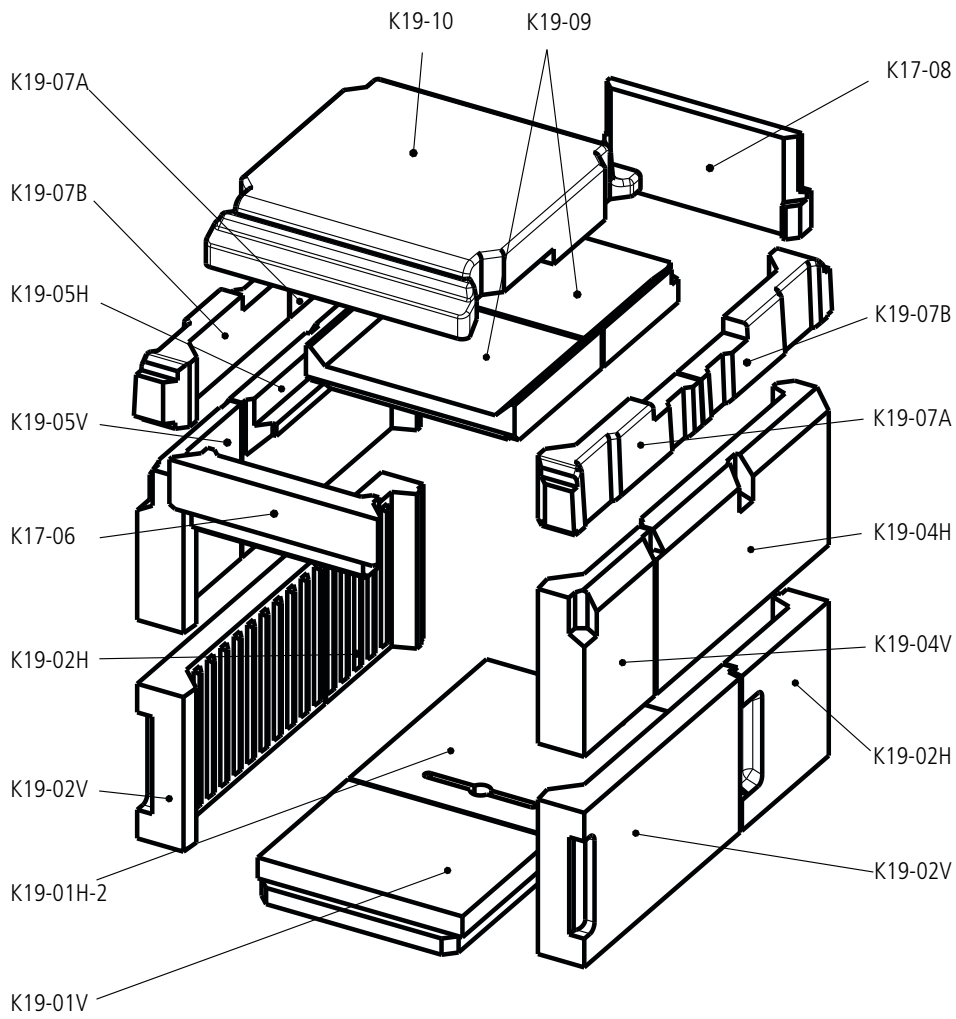
Abb. 5.9 Feuerraumauskleidung RUBIN K19.2
