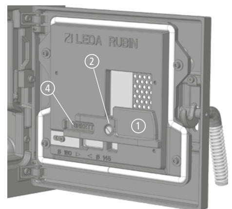
Abb. 4.14 Brennstoff-Einstellung „Braunkohlebrikett“ in der geöffneten Aschefachtür
