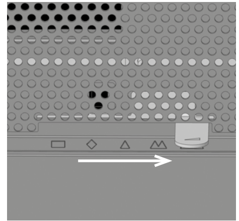
Abb. 4.20 Luftschieber ganz rechts, Anheizstellung
