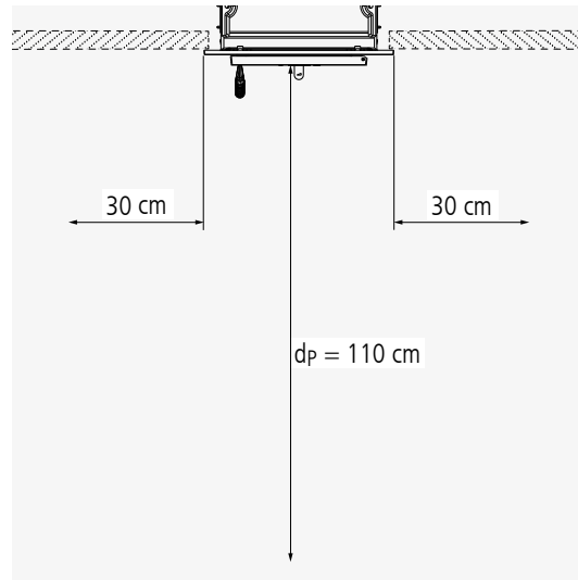
Abb. 2.3 Strahlungsbereich der Gerätefront bei RUBIN K18.2 – schematische Darstellung
