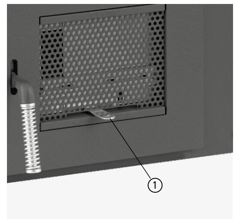
Abb. 4.3 Verbrennungsluft-Schieber in der Aschefachtür
