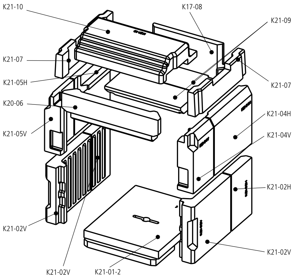
Abb. 5.12 Feuerraumauskleidung RUBIN K21.2
