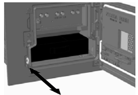
Abb. 4.12 Rüttelstange für die Rosteinrichtung, links unten neben dem Aschefach (rechts angeschlagene Aschefachtür)
