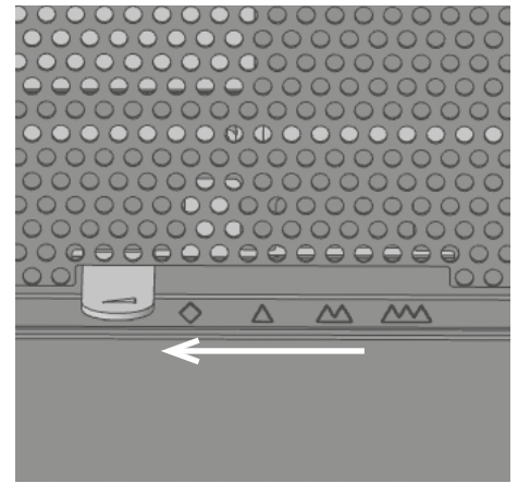
Abb. 4.30 Luftschieber ganz links, Verbrennungsluft geschlossen
