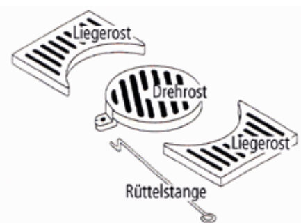
Abb. 5.7 Rosteinrichtung RUBIN
