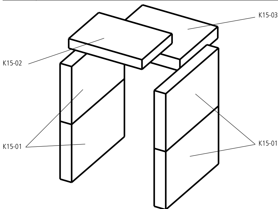
Abb. 5.1 Feuerraumauskleidung RUBIN K15.2
