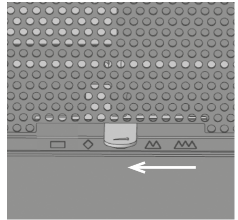
Abb. 4.11 Luftschieber ca. 1/2 geöffnet (50%), Betriebsstellung bei Nennwärmeleistung
