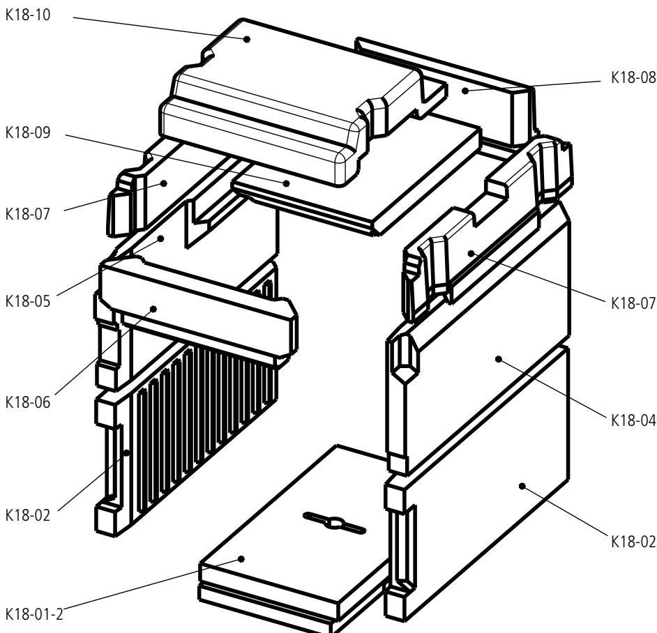
Abb. 5.6 Feuerraumauskleidung RUBIN K18.2
