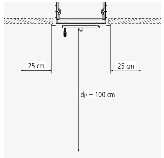
Abb. 2.5 Strahlungsbereich der Gerätefront bei RUBIN K20.2 und RUBIN K21.2 – schematische Darstellung
