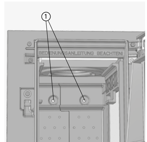
Abb. 6.1 Guss-Luftführungsplatte entnehmen
