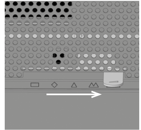
Abb. 4.28 Luftschieber ganz rechts, Anheizstellung
