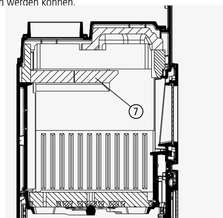
Abb. 4.40 Heizgasumlenkung
