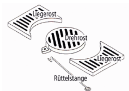
Abb. 5.8 Rosteinrichtung RUBIN
