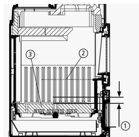
Abb. 4.38 Aschebett, Ascheniveau
