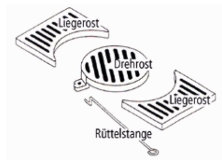
Abb. 5.3 Rosteinrichtung RUBIN
