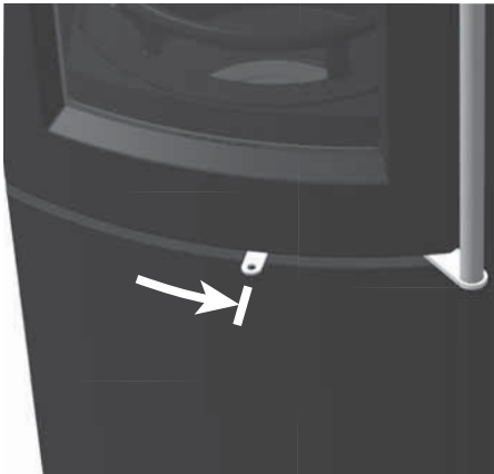
Abb. 4.24 Verbrennungslufthebel ganz rechts, Anheizstellung
