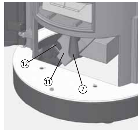
Abb. 4.36 DELTA mit LEDATRONIC: manueller Stellhebel der motorischen Luftklappe
