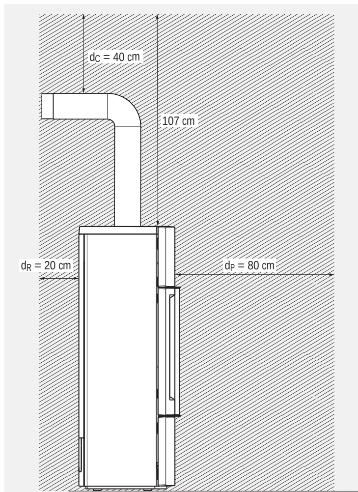
Abb. 2.5 DELTA W: Strahlungsbereich der Sichtscheibe – schematische Darstellung, Seitenansicht
