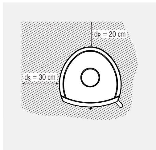
Abb. 2.7 DELTA W: Mindestabstände zu brennbaren Baustoffen oder Bauteilen
