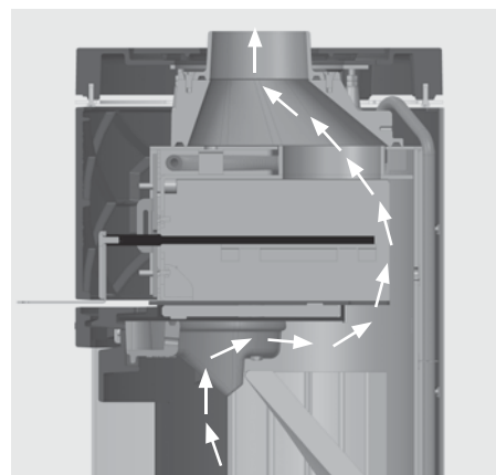
Abb. 4.13 DELTA W, Umlenkschieber heraus gezogen, Anheizstellung, Schnittdarstellung
