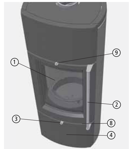
Abb. 4.1 Feuertür, Türgriff und Verbrennungslufthebel – Bedienelemente
