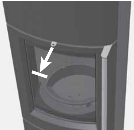
Abb. 4.25 DELTA W: Hebel oberhalb der Feuertür herausgezogen – Umlenkschieber komplett geöffnet
