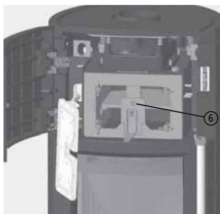
Abb. 4.51 Geöffneter Wasserwärmetauscher
