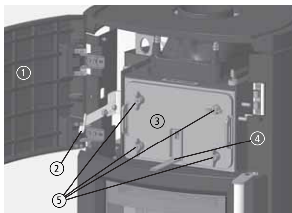
Abb. 4.50 Öffnen des Revisionsdeckels
