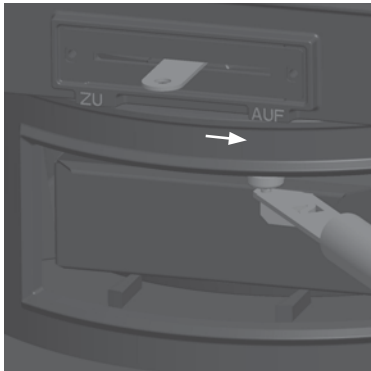
Abb. 4.23 Rüttelrost: Hebel rechts – Rost und Unterluft geöffnet
