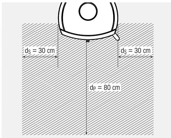
Abb. 2.4 DELTA W: Mindestabstände im Bereich der Sichtscheibe – schematische Darstellung
