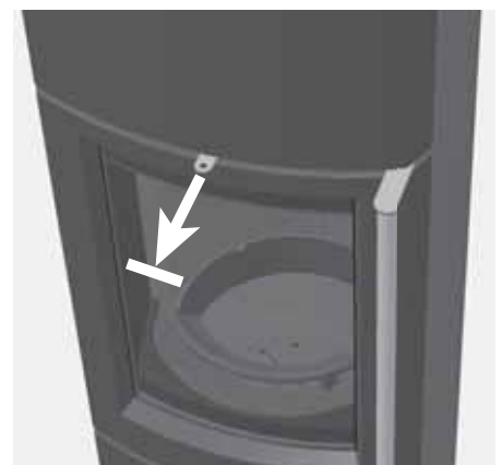
Abb. 4.22 DELTA W: Hebel oberhalb der Feuertür herausgezogen – Umlenkschieber komplett geöffnet
