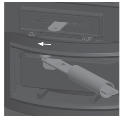
Abb. 4.16 Rüttelrost: Hebel links – Rost geschlossen
