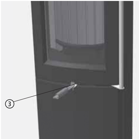
Abb. 4.7 Verbrennungslufthebel (hier mit Bediengriff)
