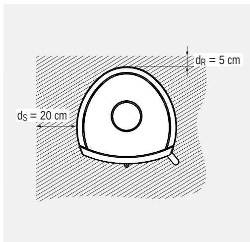
Abb. 2.6 DELTA plus (ohne Wassertechnik): Mindestabstände zu brennbaren Baustoffen oder Bauteilen
