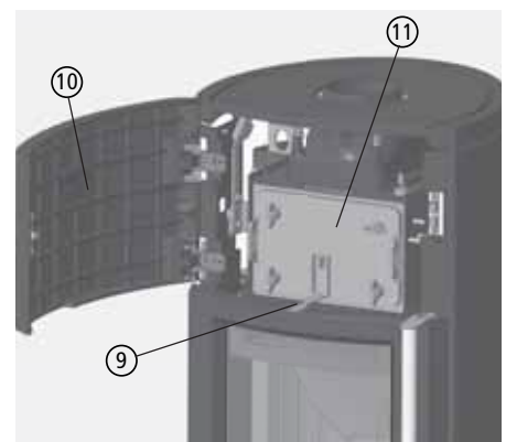
Abb. 4.3 Revisionstür bei DELTA W
