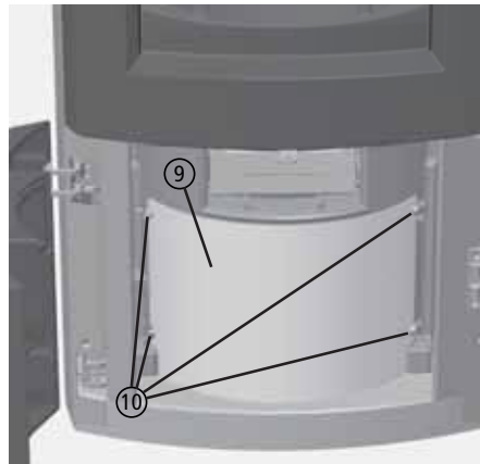
Abb. 4.35 DELTA mit LEDATRONIC: Edelstahlabdeckung vor der motorischen Luftklappe
