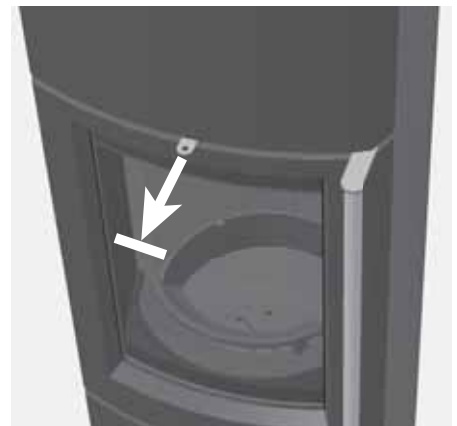
Abb. 4.15 DELTA W: Hebel oberhalb der Feuertür herausgezogen – Umlenkschieber komplett geöffnet
