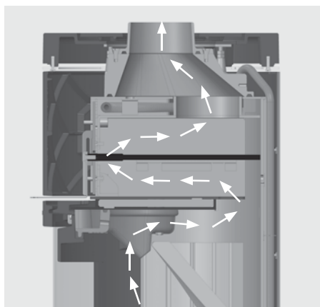
Abb. 4.12 DELTA W, Umlenkschieber hinein geschoben, Betriebsstellung, Schnittdarstellung
