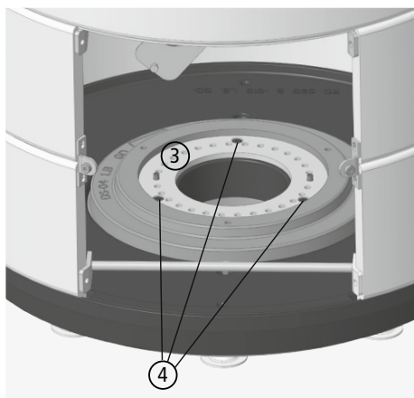
Afb. 3.27 Verwijderen van de stelschijf voor de zijdelingse aanslagen
