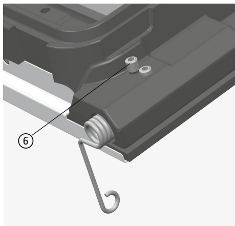
Afb. 3.9 deurveer borgen
