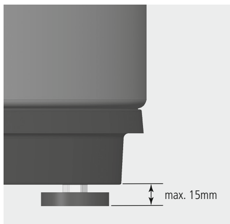
Afb. 3.1 Stelvoetjes onder de bodem van het apparaat
