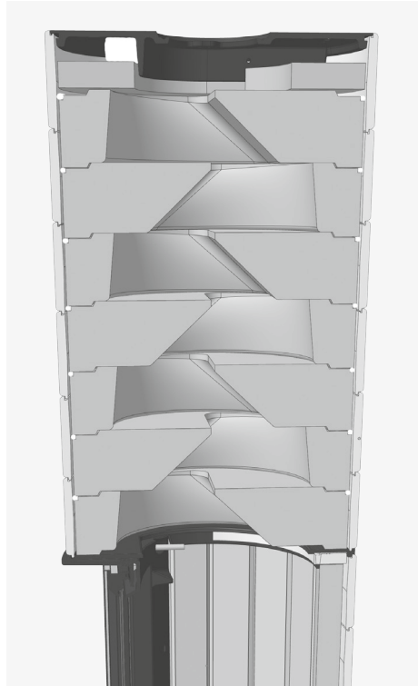
Afb. 3.29 Opbouw van het opzetstuk
