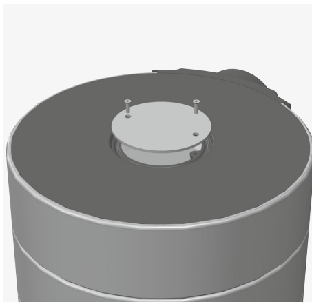
Afb. 3.31 Blinddeksel monteren
