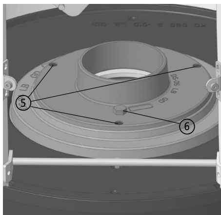
Afb. 3.25 Montage van het bovengedeelte van de draaiconsole
