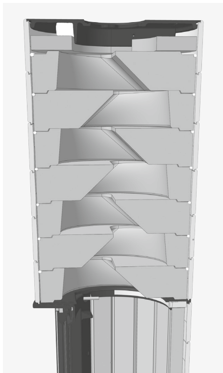
Afb. 4.8 Verwarmingsgasweg in het opzetstuk
