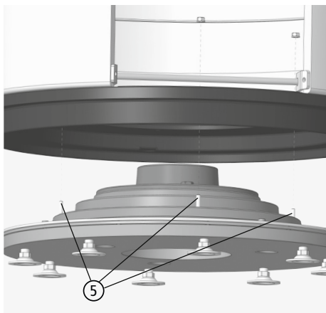
Afb. 3.17 Stelschroef met bovengedeelte van de draaiconsole
