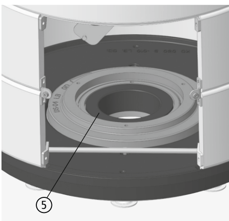
Afb. 3.28 Verbrandingsluchtleiding, van onder
