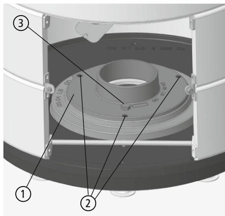
Afb. 3.22 Bovenste deel van de draaiconsole
