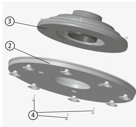
Afb. 3.16 Draaiconsole met bodemplaat en bovengedeelte
