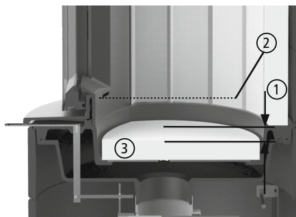
Afb. 4.7 Asbed, ashoogte
