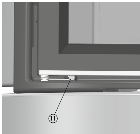
Afb. 3.11 deurveer spannen
