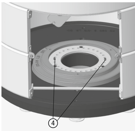
Afb. 3.23 Stoppen, het instellen van de linker en rechter eindaanslagen
