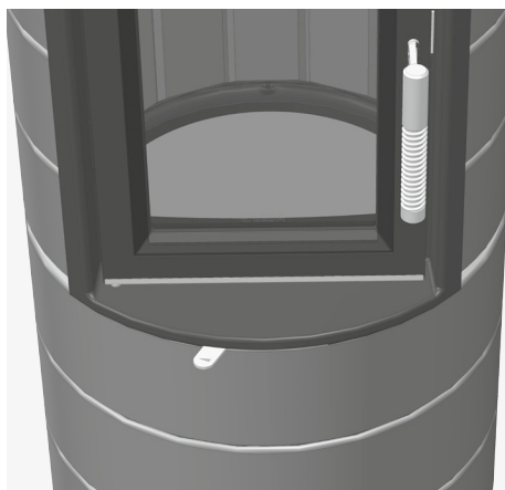
Afb. 4.3 verbrandingsluchtschuif, links, volledig gesloten
