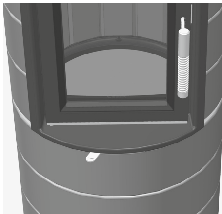
Afb. 4.6 verbrandingsluchtschuif, links, volledig gesloten
