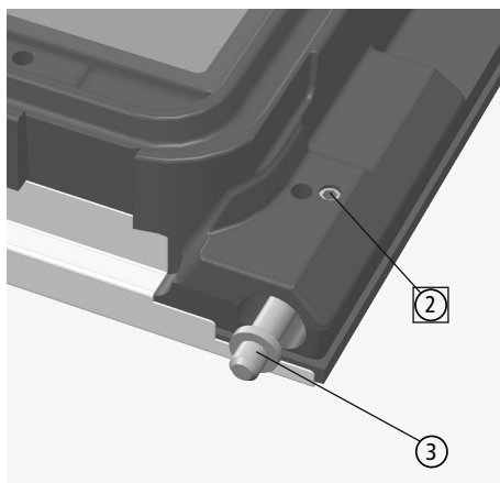
Afb. 3.7 onderste scharnierpen verwijderen
