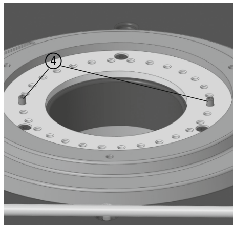
Afb. 3.24 Aanslagpennen, instellen van de linker en rechter eindaanslag
